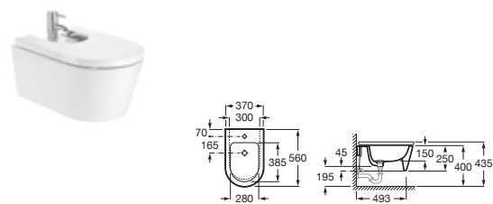
Bidet podwieszany Round
