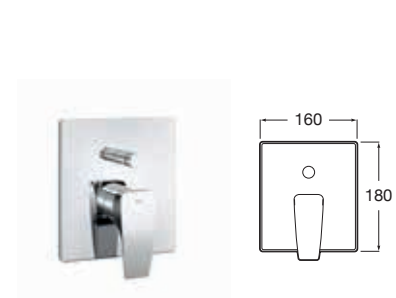
Element zewn. do ROCABOX wannowo-natryskowy (Do kompletacji z elementem podtynkowym Rocabox str. 176)
