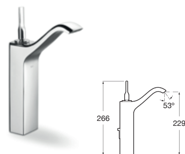
Jednouchwytywa bateria umywalkowa sztorcowa wysoka
