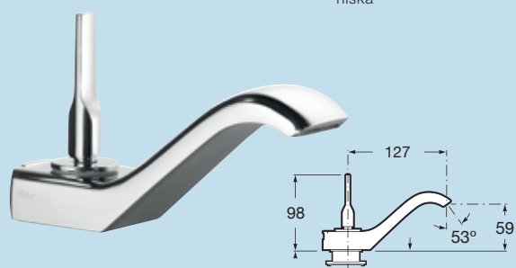
Jednouchwytywa bateria umywalkowa sztorcowa niska
