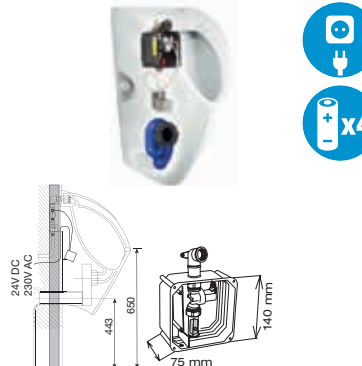
Pisuar z zaworem radarowym
