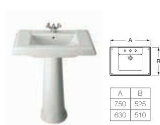
Umywalka ścienna / postument
