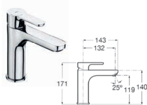
Bateria umywalkowa średnia z uchwytem XL z COLD START
