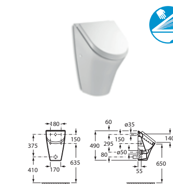
Pisuar z pokrywą wolnoopadającą
