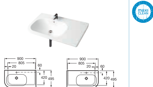
Umywalka ścienna lewa i prawa
