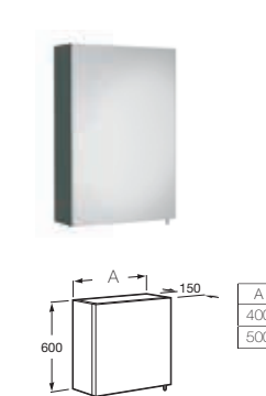
Szafka Luna z lustrem
