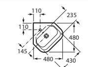
Umywalka narożna lewa
