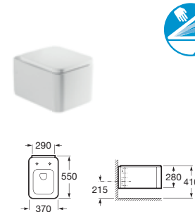
Miska WC podwieszana
