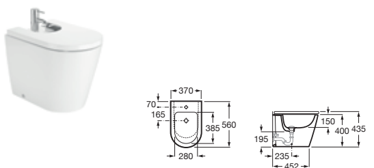
Bidet stojący Round
