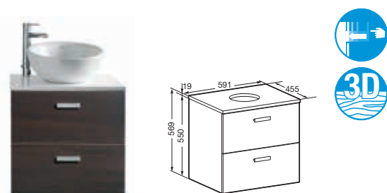
Szafka z blatem z 2 szufladami pod umywalki nablutowe
