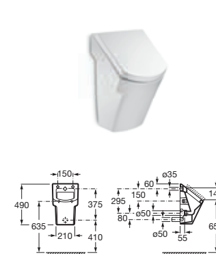
Pisuar z pokrywą wolnoopadającą
