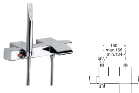
Termostaticzna bateria wannowo-natryskowa z zestawem natryskowym ze stelażem
