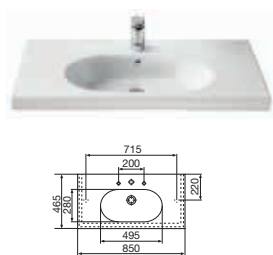
Umywalka meblowa z blatem
