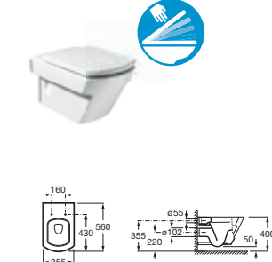
Miska WC podwieszana
