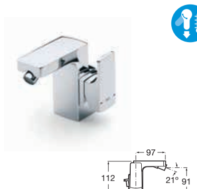
Jednouchwytowa bateria bidetowa sztorcowa, uchwyt boczny
