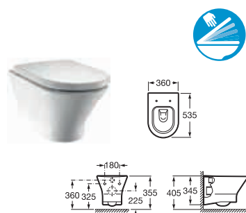
Miska WC podwieszana Rimless
