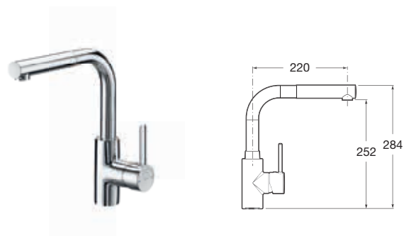
Bateria zlewozmywakowa z wyciąganą i obrotową wylewką
