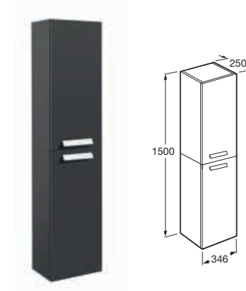
Kolumna wysoka obustronna z 4 półkami
