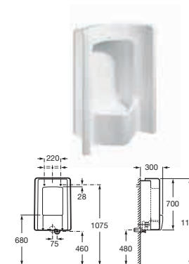
Pisuar ze ściankami bocznymi
