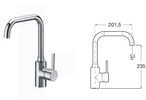
Bateria zlewozmywakowa z obrotową wylewką SQUARE
