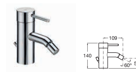
Bateria bidetowa bez COLD START z korkiem automatycznym
