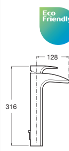
Jednouchwytywa bateria umywalkowa sztorcowa wysoka
