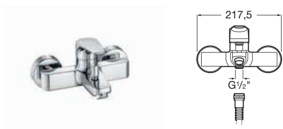
Bateria wannowo-natryskowa ścienna
