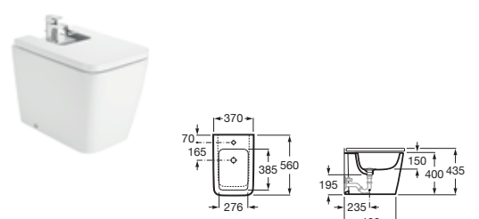
Bidet stojący Square
