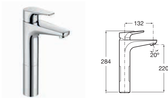
Bateria umywalkowa wysoka z COLD START
