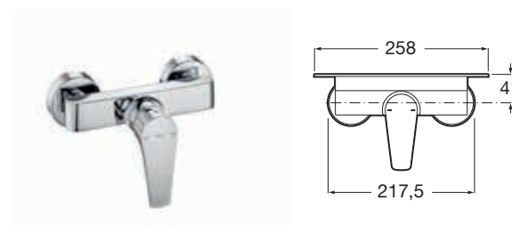
Bateria natryskowa ścienna
