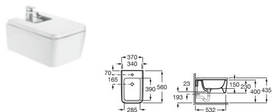
Bidet podwieszany Square
